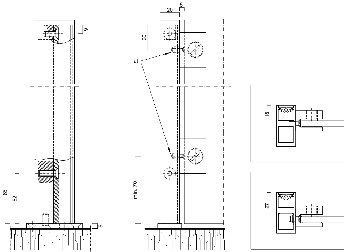
Glashalter 414.5531.XXX Max. Glasmaße: Länge 1.400 mm, Höhe 600 mm.
