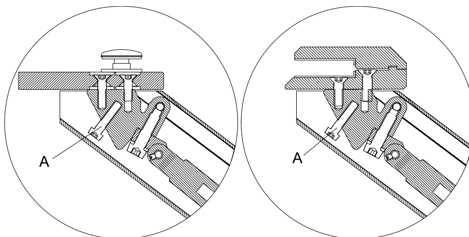
Zahlplatte mit Punkthalterung (links) bzw. Glasklammer (rechts) A = Stellschraube zur waagerechten Ausrichtung der Zahlplatte
